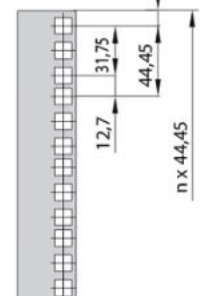
19"-Profilschiene
