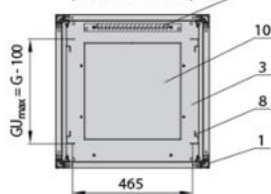
Schnitt C-C (Schrantiefe 600 mm)
